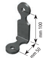
Art. 343 Staffa di collegamento tra pannello e muretto spessore mm 4 Foro mm 12 spessore mm 6 Foro mm 13 Grezzo
