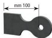
Art. BL 280 Staffa di fissaggio su colonna e pannello in lamiera Dim. mm 120x40 spessore mm 4 Foro mm 12 spessore mm 6 Foro mm 13 Grezzo
