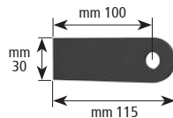
Art. BL 319 Staffa di fissaggio su colonna e pannello in lamiera Dim. mm 115x30 spessore mm 4 Foro mm 12 spessore mm 6 Foro mm 13 Grezzo
